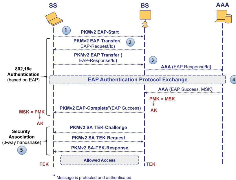
Fig. 6. IEEE 802.16e message flow
