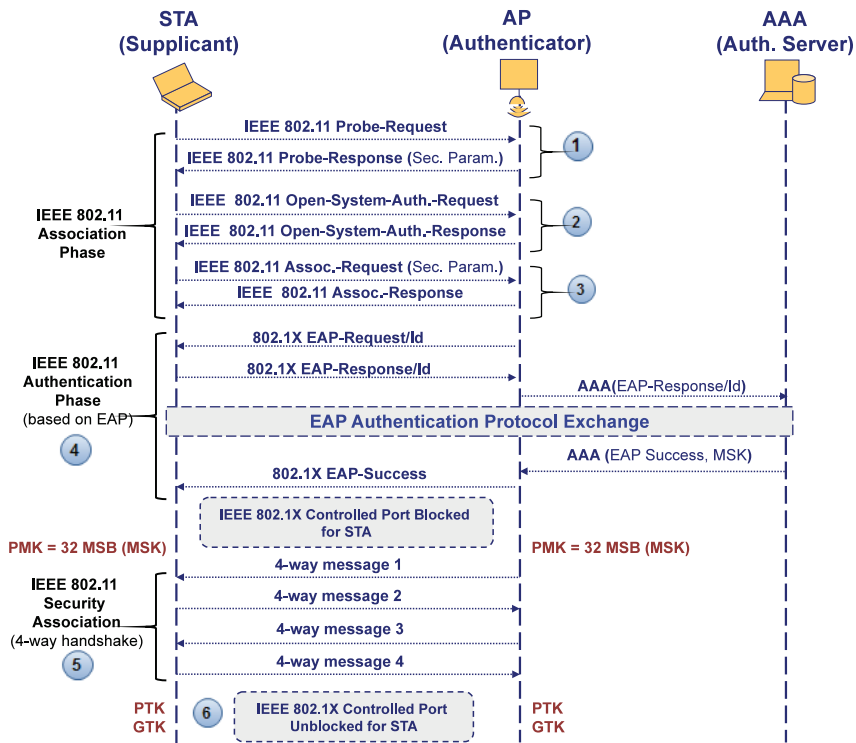
Fig. 5. IEEE 802.11 message flow
